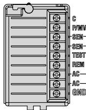
Module de puissance du programmeur Hunter (standard)
